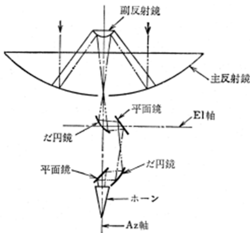
図 5.2.10 4 回反射集束ビーム給電カセグレンアンテナ
